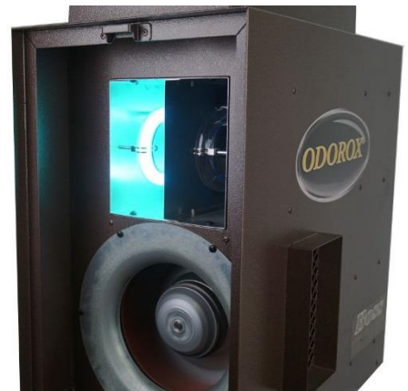
Boss Geruchsneutralisator, Seitenansicht ohne Abdeckung
